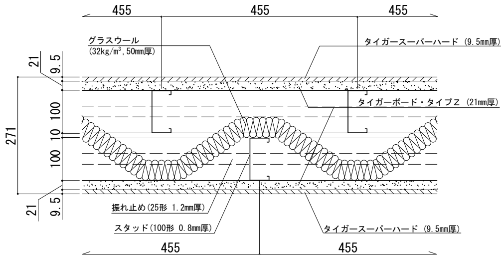
水平断面図（「タイガードリーミィ・65」遮音測定時（S-271-25参照）の壁構造）
