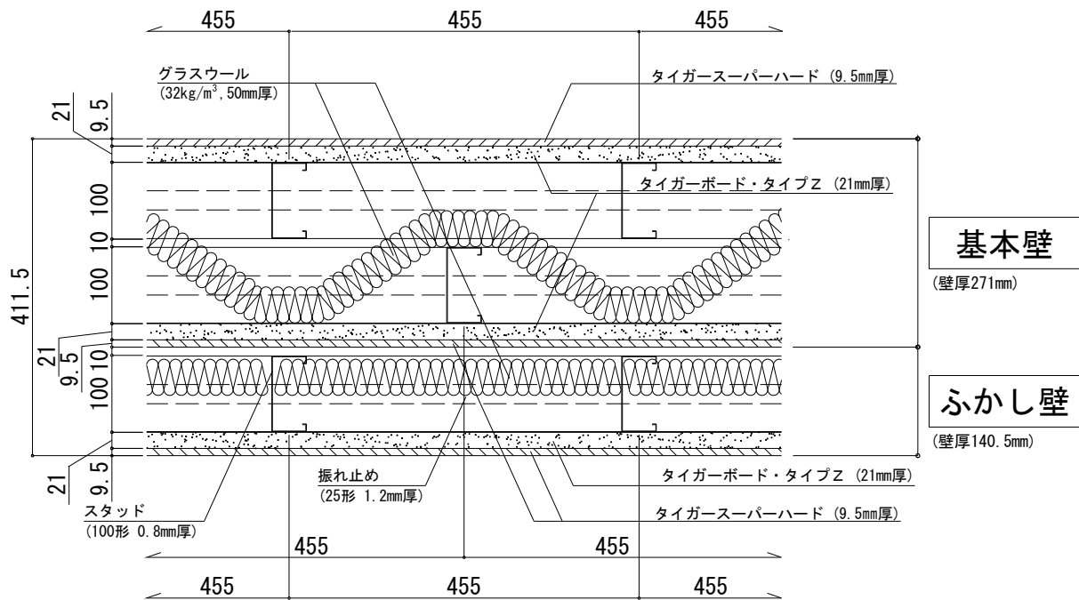
水平断面図（「タイガードリーミィ・75」遮音測定時（S-271-26参照）の壁構造）
