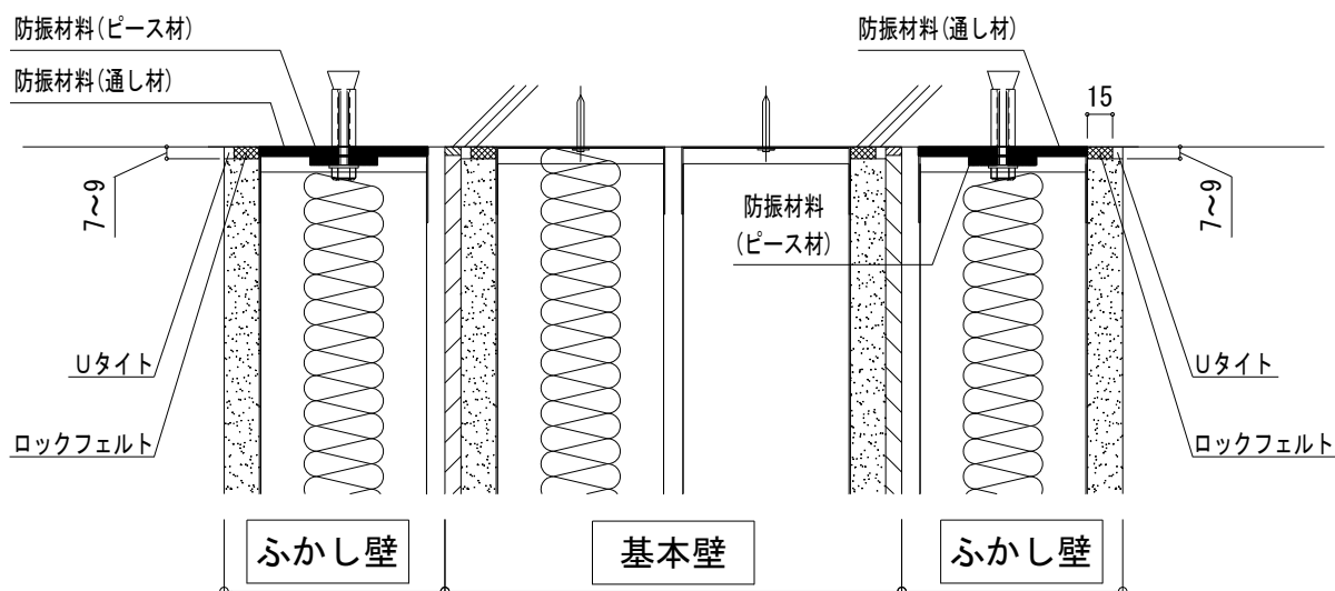
<タイガードリーミィ・75のスラブ下の納まり例>
