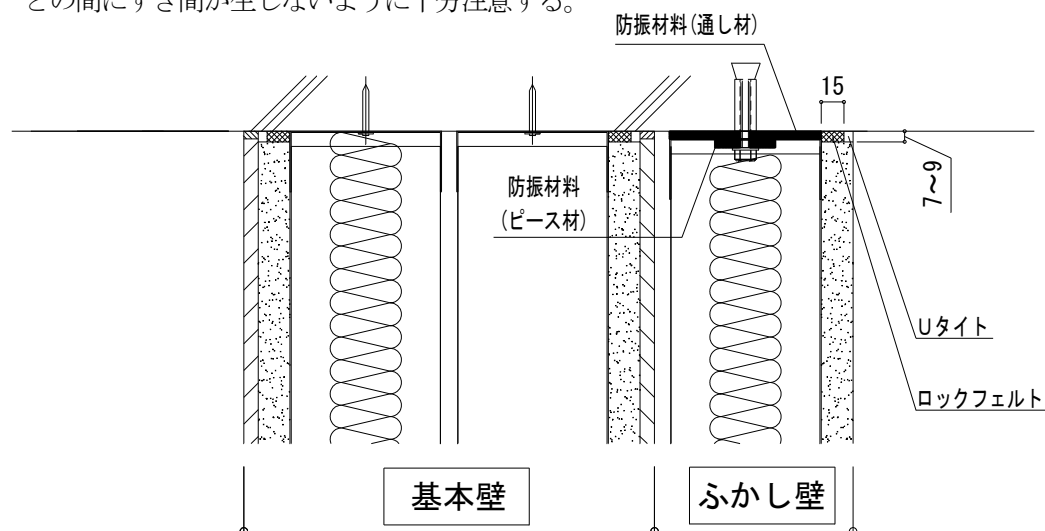
<タイガードリーミィ・75のスラブ下の納まり例>
